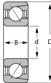
Vinkelkontaktlager, enradigt
