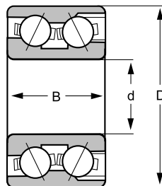
Vinkelkontaktlager, tvåradigt
