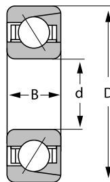
Vinkelkontaktlager, enradigt
